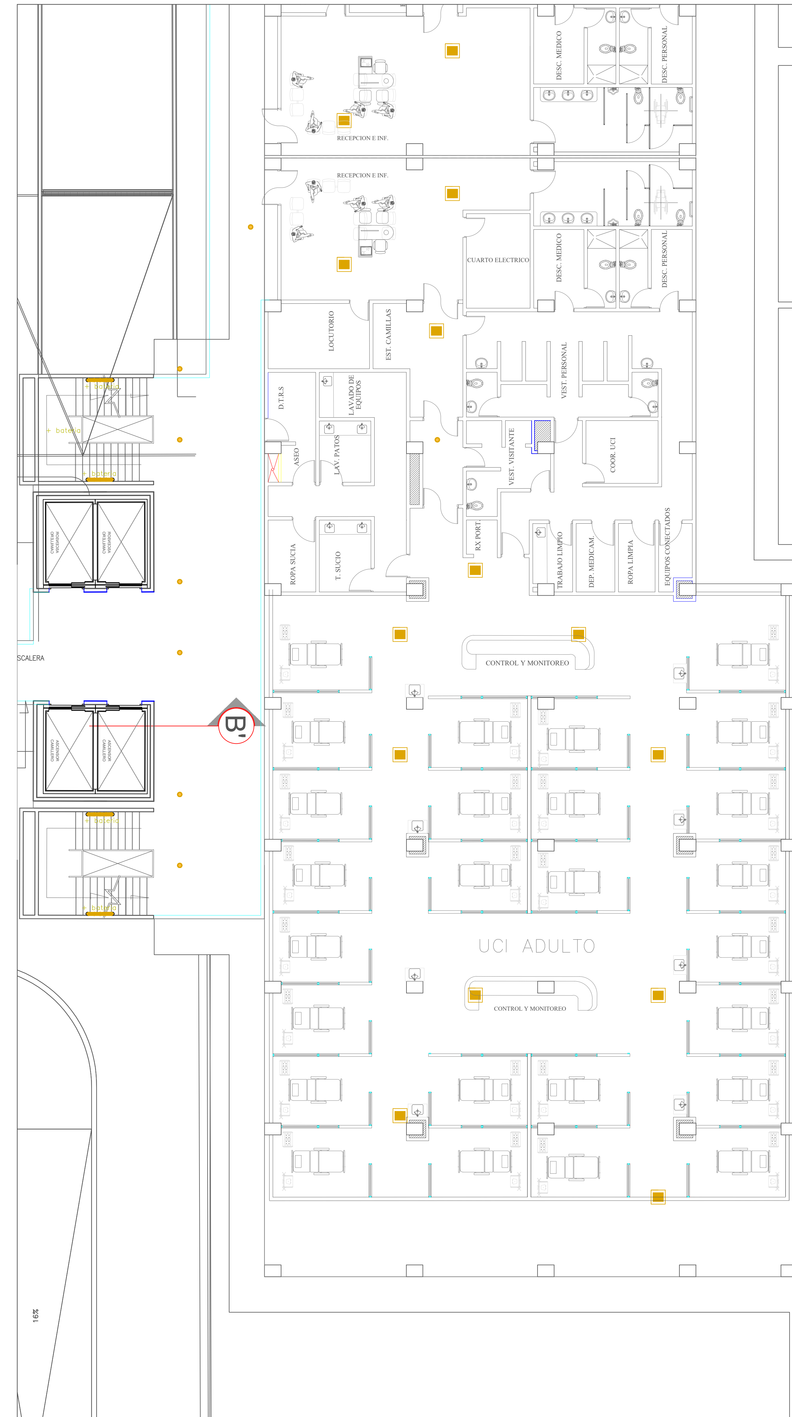
ILUMINACION PISO2-PARTEB
